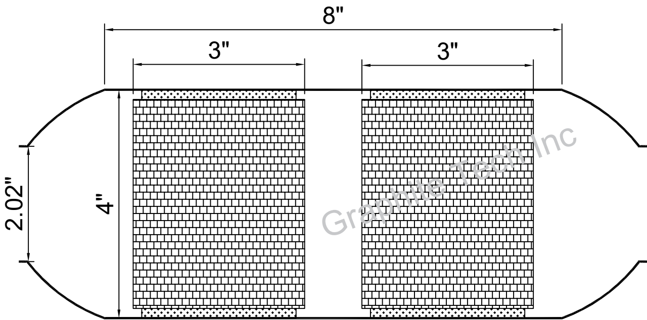
Part No : G4-2-8-3+3
