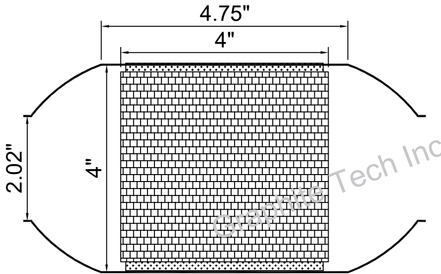
Part No : G4-2-4.75-4
