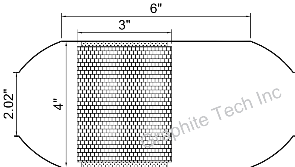
Part No : G4-2-6-3
