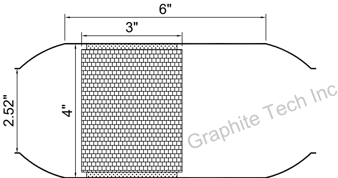
Part No : G4-2.5-6-3
