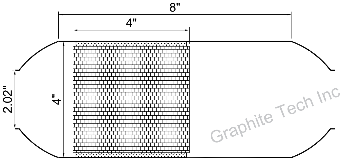
Part No : G4-2-8-4
