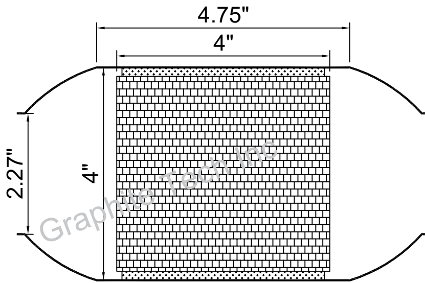
Part No : G4-2.25-4.75-4
